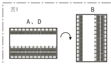
规格尺寸为 A、B、C、D 型接线图
