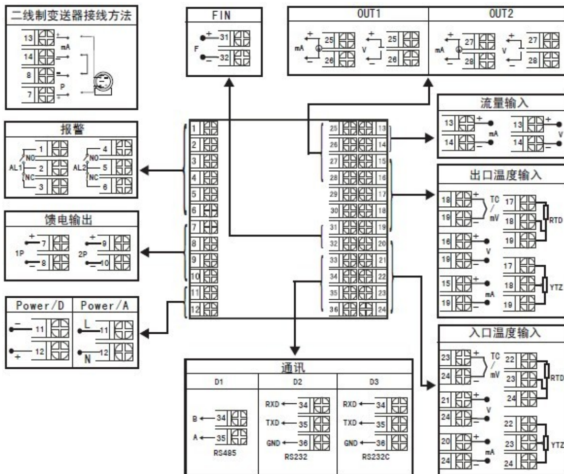
规格尺寸为 A、B、C、D 型接线图
